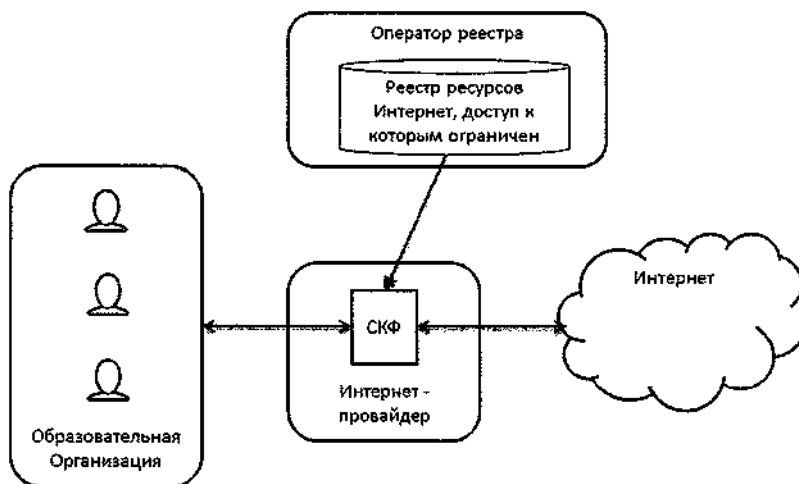
Рисунок 4. Схема работы контент-фильтрации при размещении у Интернет-провайдера
